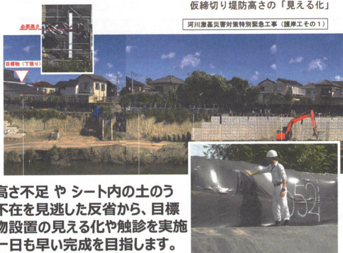
仮締切り堤防高さの「見える化」
